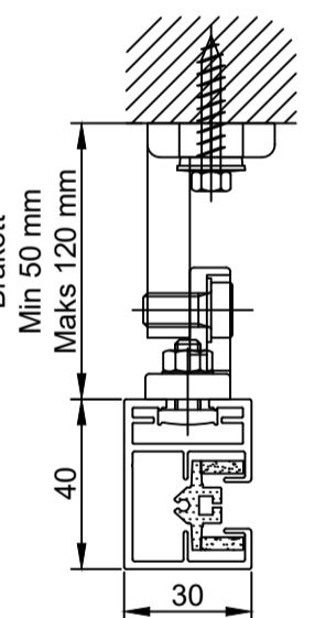
Styreskinne 40x30 mm på brakett
