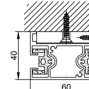
Styreskinne 40x60 mm dobbel
