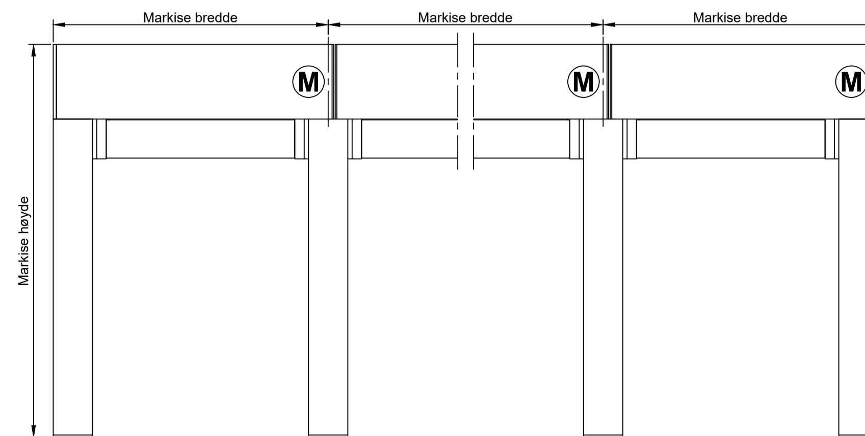
Installasjons muligheter: i serie; motor side høyre Motor side alltid på samme side i en serie
