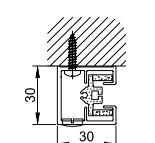
Styreskinne 30x30 mm
