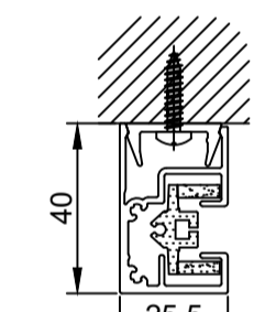
Klikk skinne 40x25,5 mm
