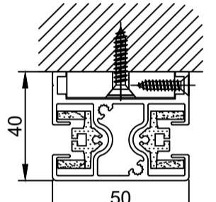
Styreskinne 40x50 mm dobbel
