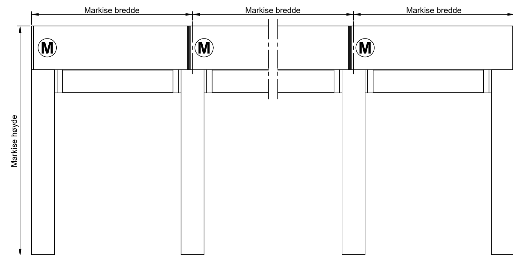
Installasjons muligheter: i serie; motor side venstre Motor side alltid på samme side i en serie
